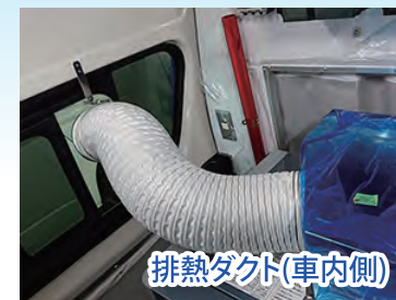
SHR-40Pエアリアル設置例
